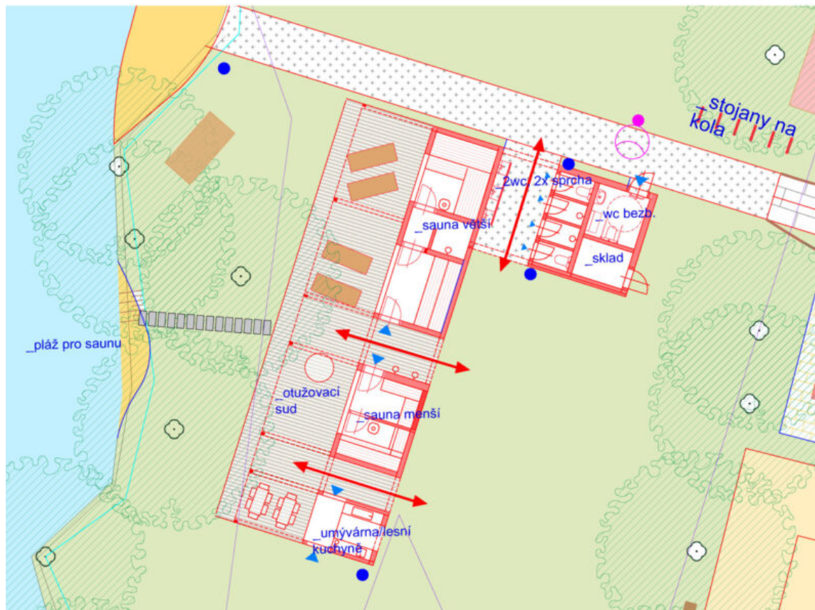
Půdorys jižního "saunového" objektu
