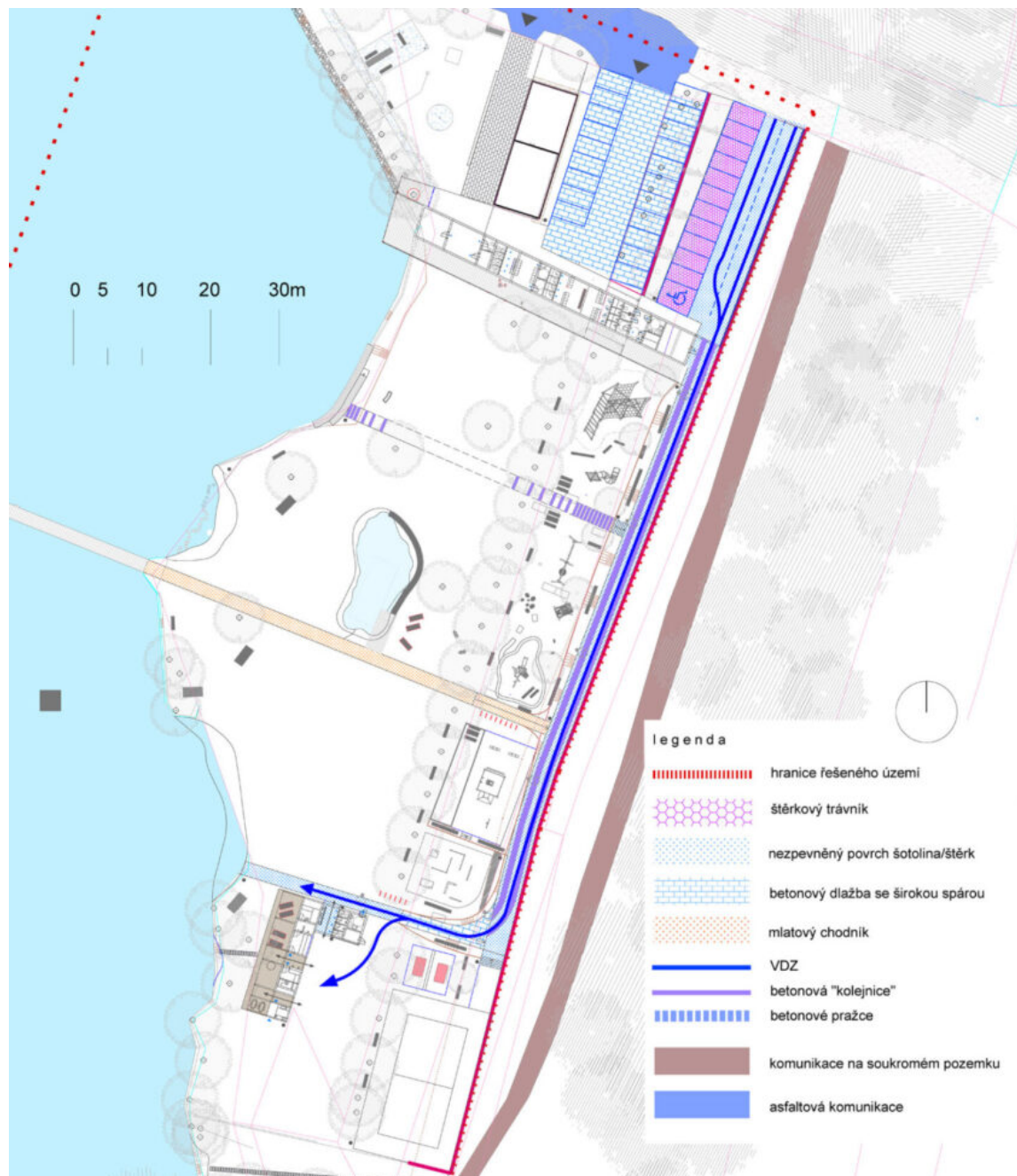
Situace dopravy v areálu
